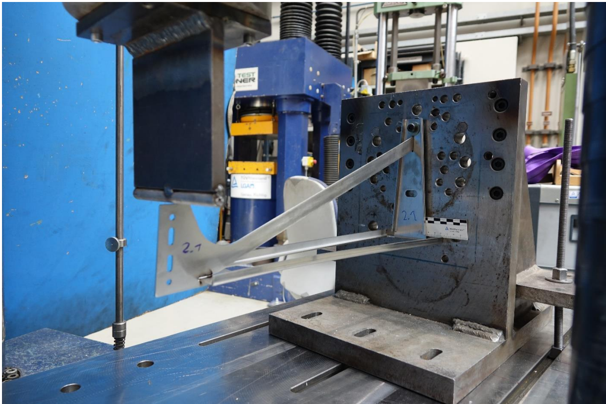
Bild 5. Winkel 2.1 nach der Belastung in der Prüfmaschine.
