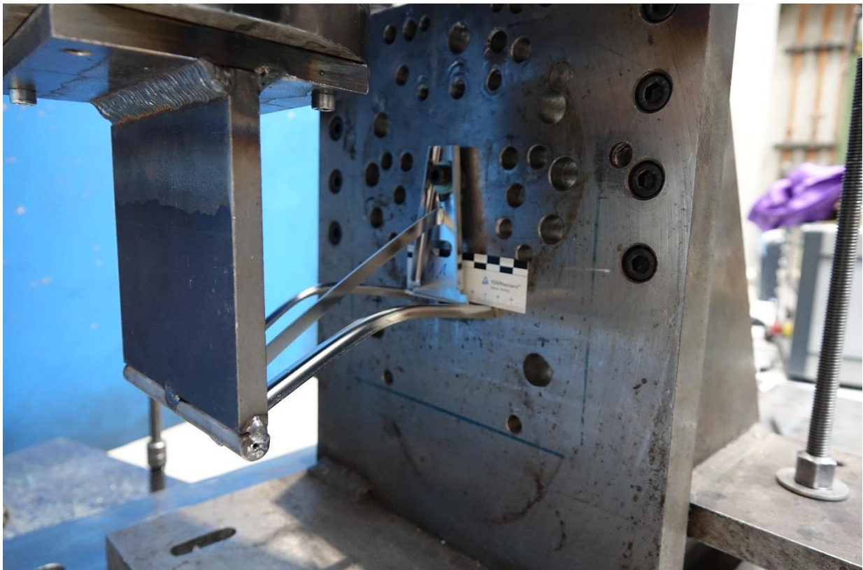
Bild 2. Winkel 1.1 nach der Belastung in der Prüfmaschine.
